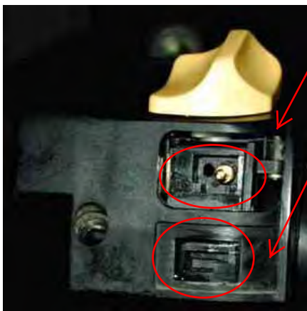
Blinkerrücksteller wieder anschrauben Blinkerbetätigung auch festschrauben
