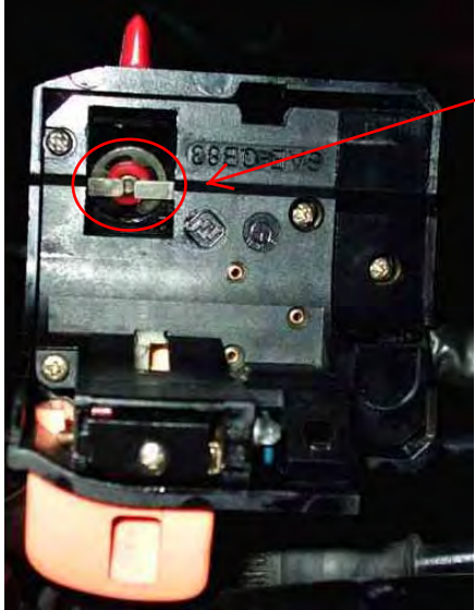
Wiedereinsetzen des roten Hebels Sicherungsscheibe nicht vergessen!
