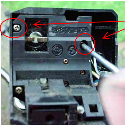
Lösen der zwei Schrauben innerer Deckel
