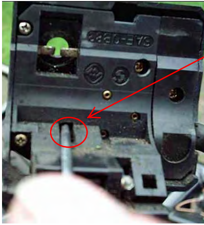
Lösen der Schraube Lichtschieber
